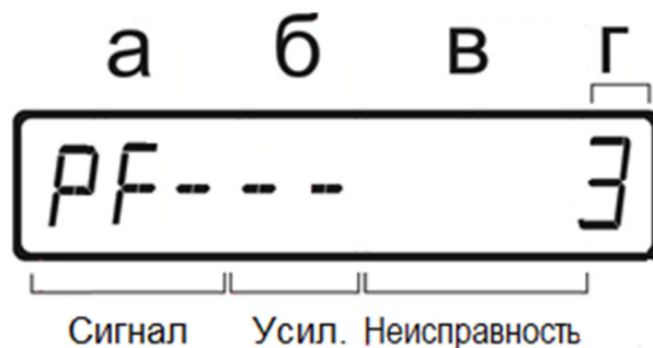
Рисунок 2.4 - Отображение на дисплее прибора контроля информации об отклонении напряжения питания ИПДЛ от допустимого
