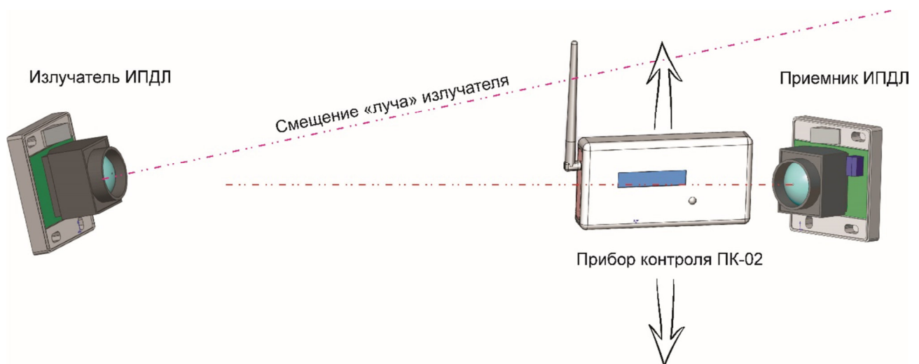
Рисунок 2.1 - Размещение прибора контроля ПК-02 при работе в режиме «Детектор поля ИПДЛ»
